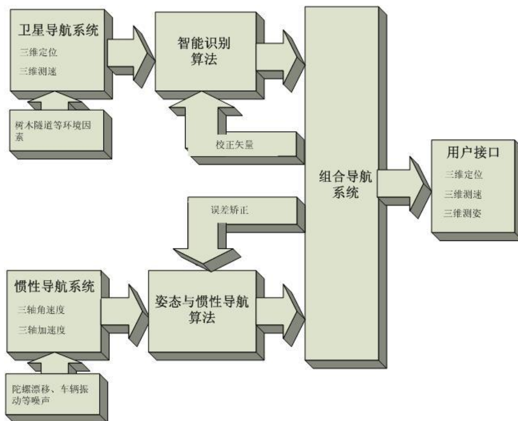
图 3: SKM3507MR-40MXT 设计原理框图/Design diagram
