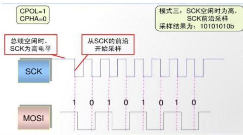
图 6-4 CPOL=1 CPHA=0
