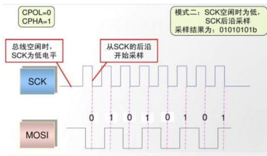
图 6-3 CPOL=0 CPHA=1
