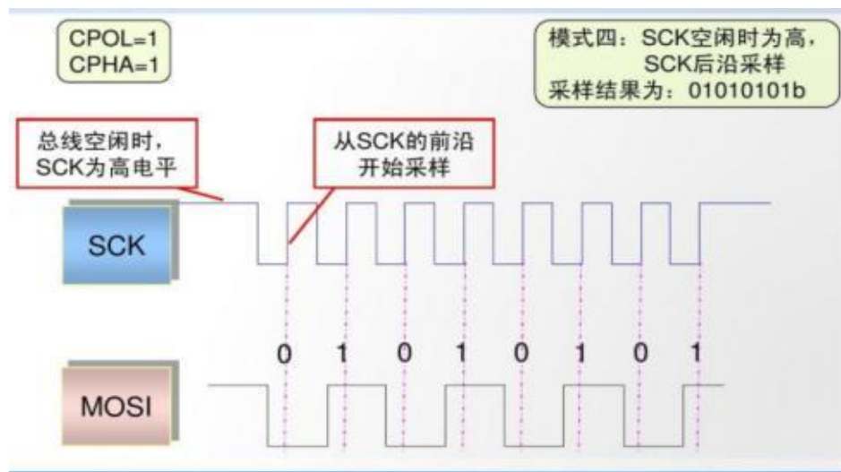
图 6-5 CPOL=1 CPHA=1
