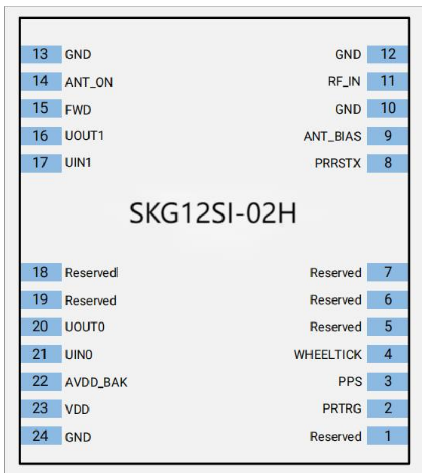
图 3 SKG12SI-02H 引脚分布
