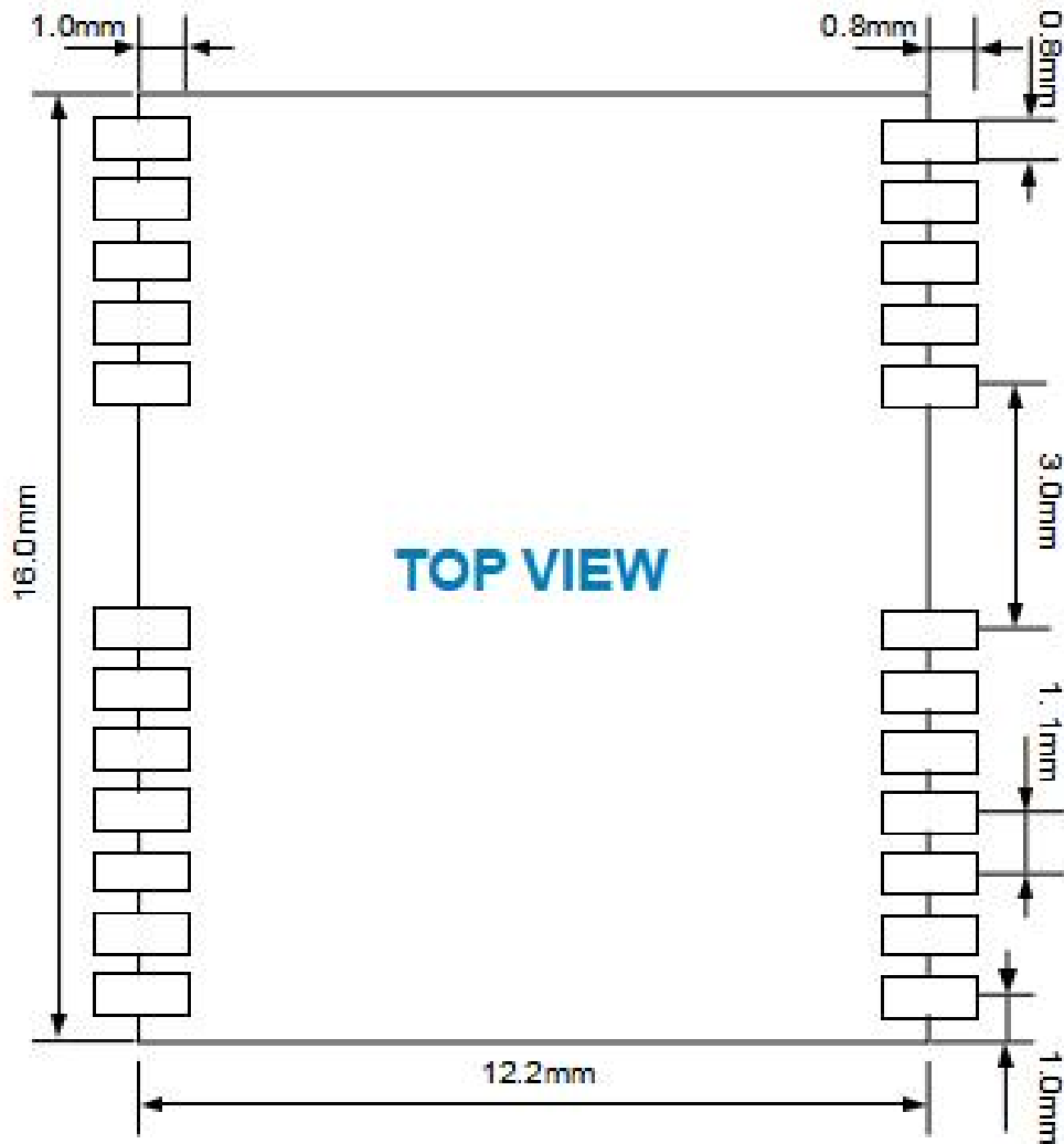
图 9 SKG12SI-02H 封装参考
