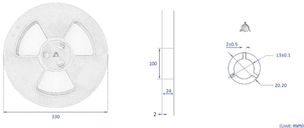
图 12 卷盘
