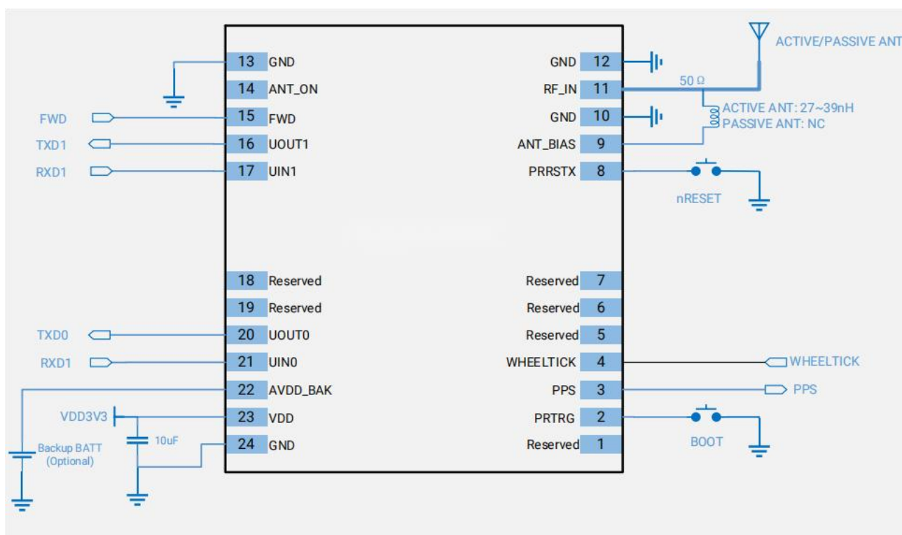
图 8 参考设计原理图
