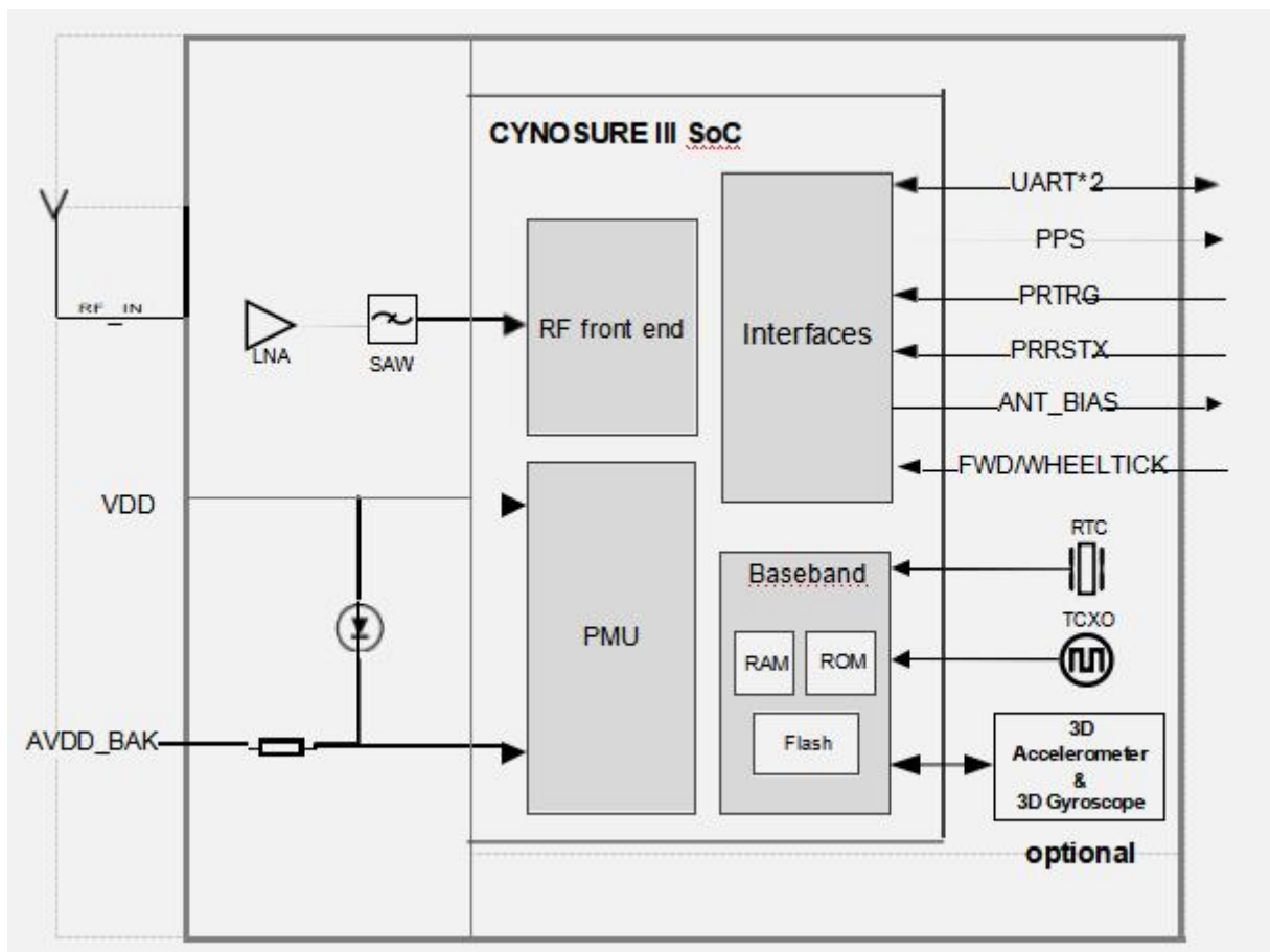
图 2 系统框图
